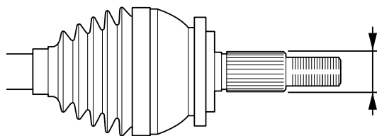
Illustration 1 : Mesurer le diamètre extérieur de l'arbre d'essieu pour identifier le bon roulement de roue.
