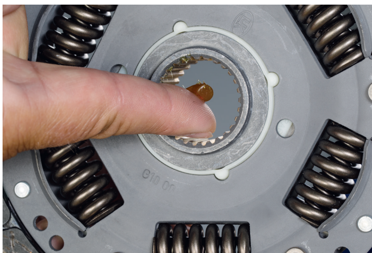
Photo 1: Graissage de la denture du moyeu
